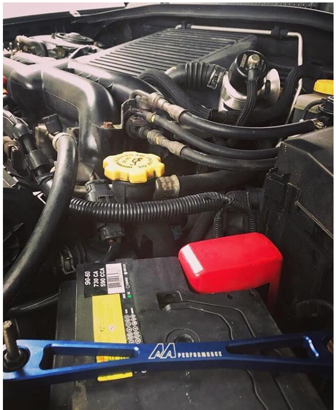
2- Support à batterie installé sur un Subaru legacy gt 2007
