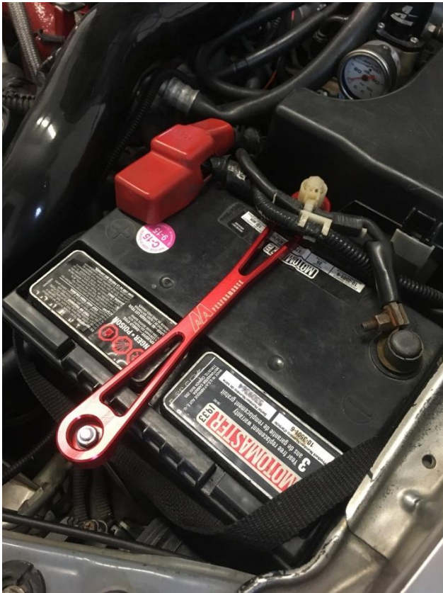
1- Support à batterie installé sur un Subaru sti 2006 avec une batterie « aftermarket »
